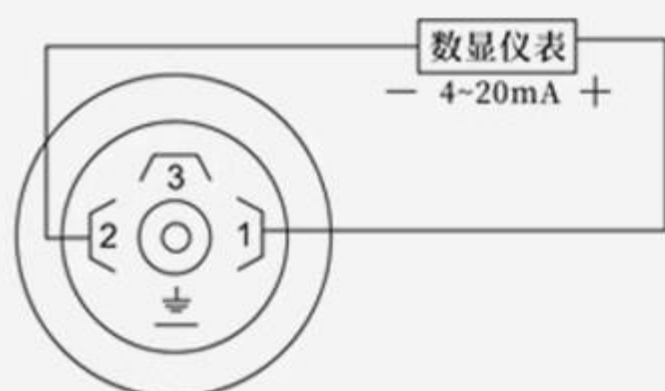
ELE-301、801、806 二线制带DC24V馈电
