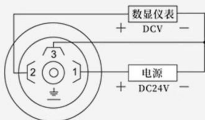
ELE-301、801、806 三线制电压输出
