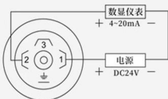
ELE-301、801、806 二线制需附加电源输出
